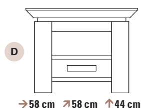
Maatvoering buitenmaten S4
